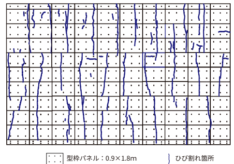
標準養生後のひび割れマップ
