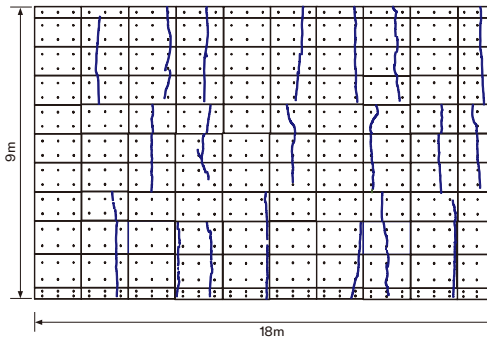
養生テープ処理後のひび割れマップ
